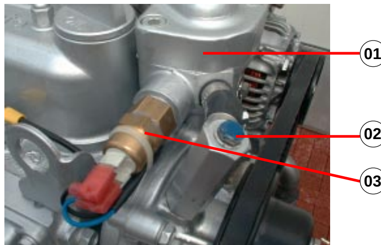
Temperaturschalter am Thermostatgehäuse
