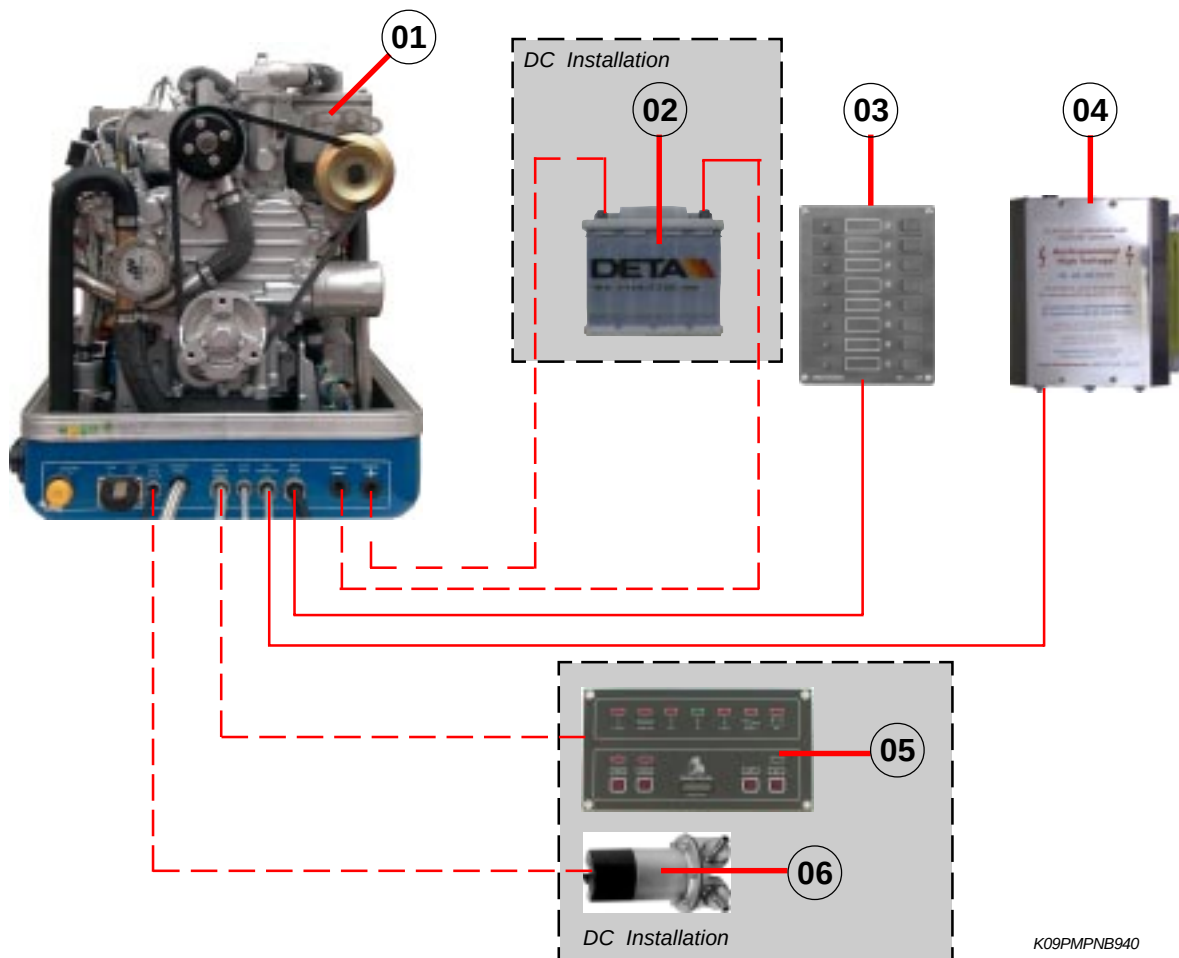
Anschlußplan Beispiel Panda 8000
