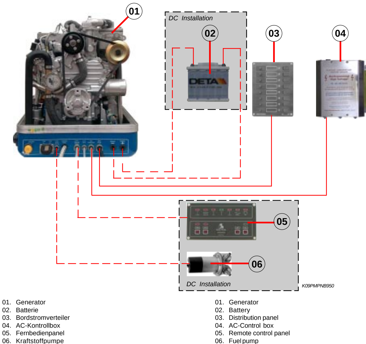
Anschlußplan Beispiel Panda 8000
