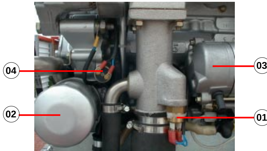
Temperaturschalter am Auspuff / Öldruckschalter
