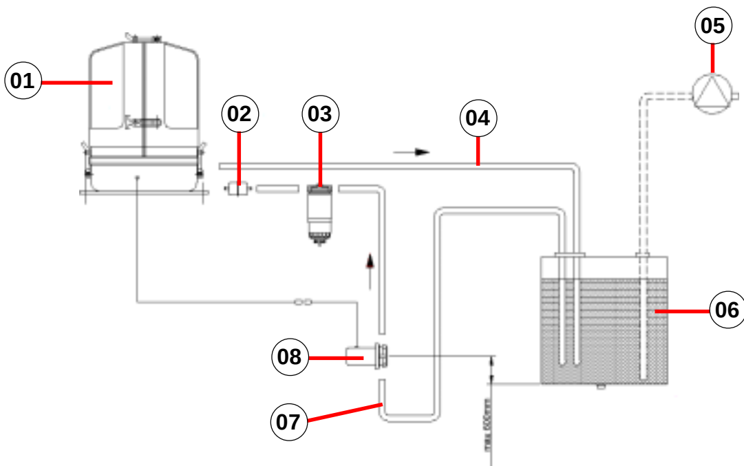
Anschluß an das Kraftstoffsystm
