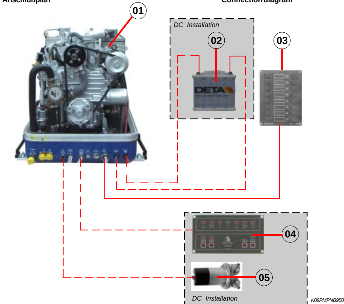
Anschlußplan
