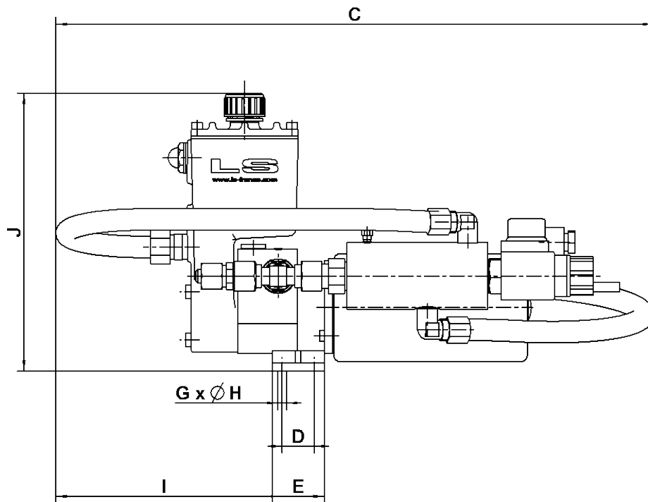
Ensemble linéaire Linear drive 32 ST16 BP - 40 T 254 BP
