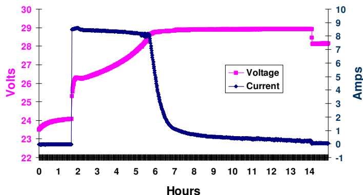
Exemple de courbe de la charge d'une batterie enregistrée avec un logiciel BMV602 et VEBat
