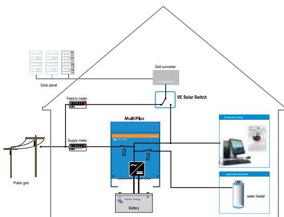
Schéma 3. Système à deux compteurs avec MultiPlus et Interrupteur Solaire
