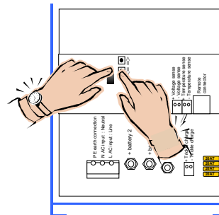
Paramétrage de la tension 'Float'
