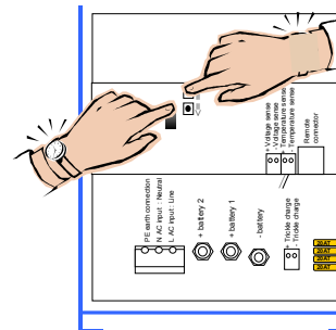
Paramétrage de la tension d'absorption
