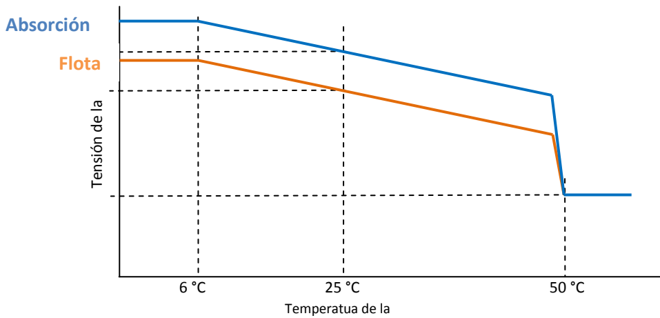
Figura 1: curva de compensación de temperatura
