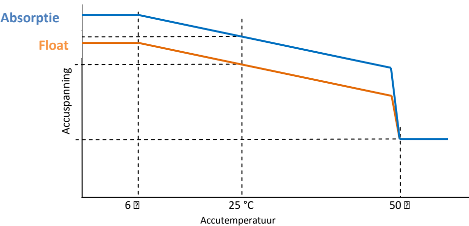
Afbeelding 1: temperatuurcompensatiecurve
